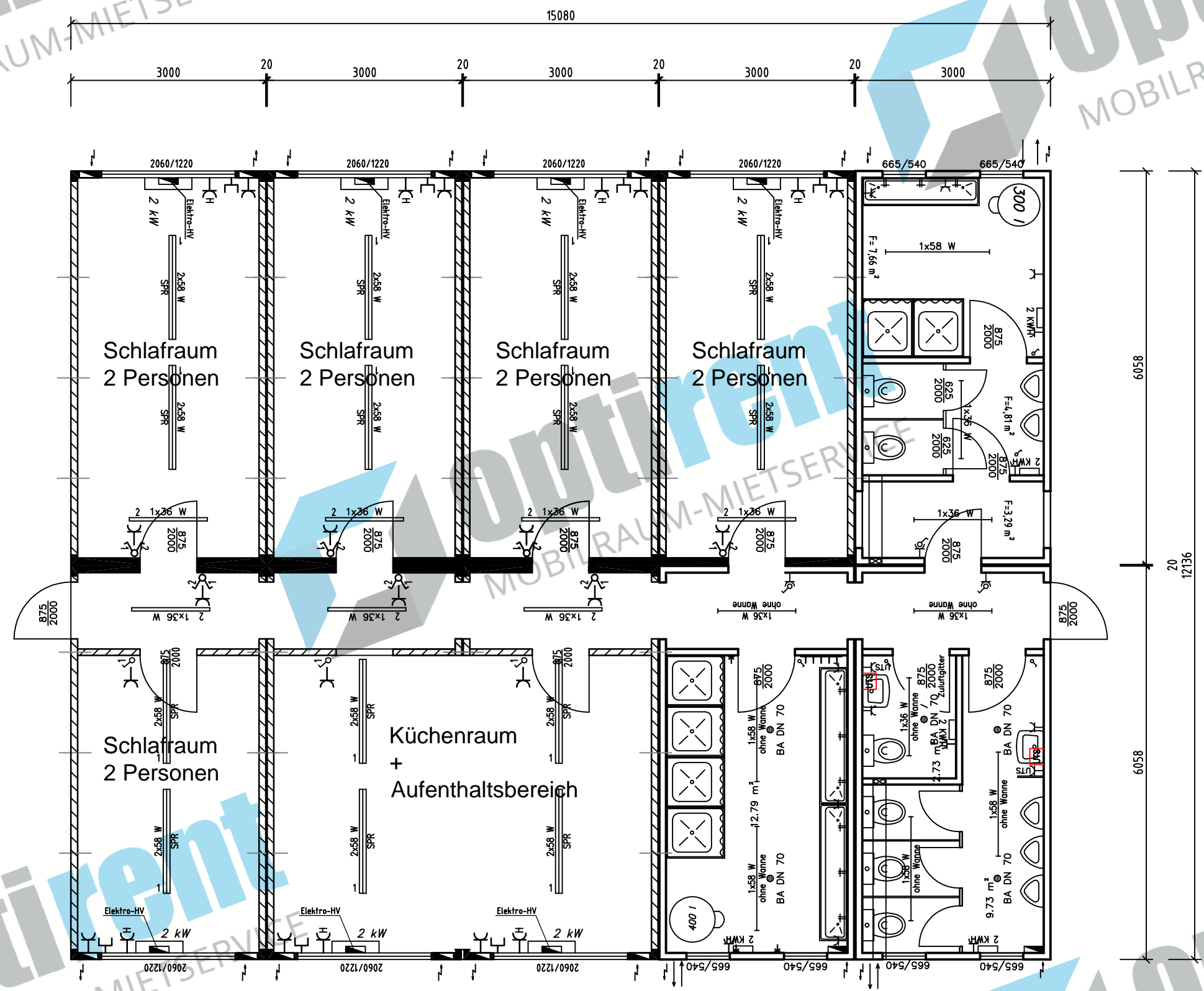
Wohncontaineranlage für 10 Personen Damen- und Herren Sanitärbereiche getrennt Inkl. Küchen- und Aufenthaltsraum
